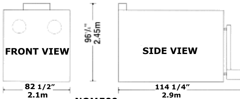
NOM 500
