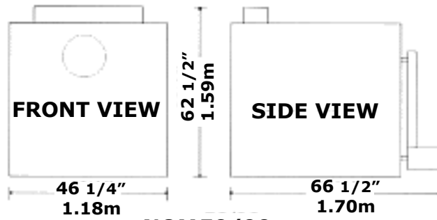
NOM 50/90
