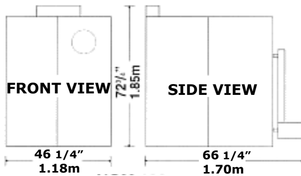
NOM 120
